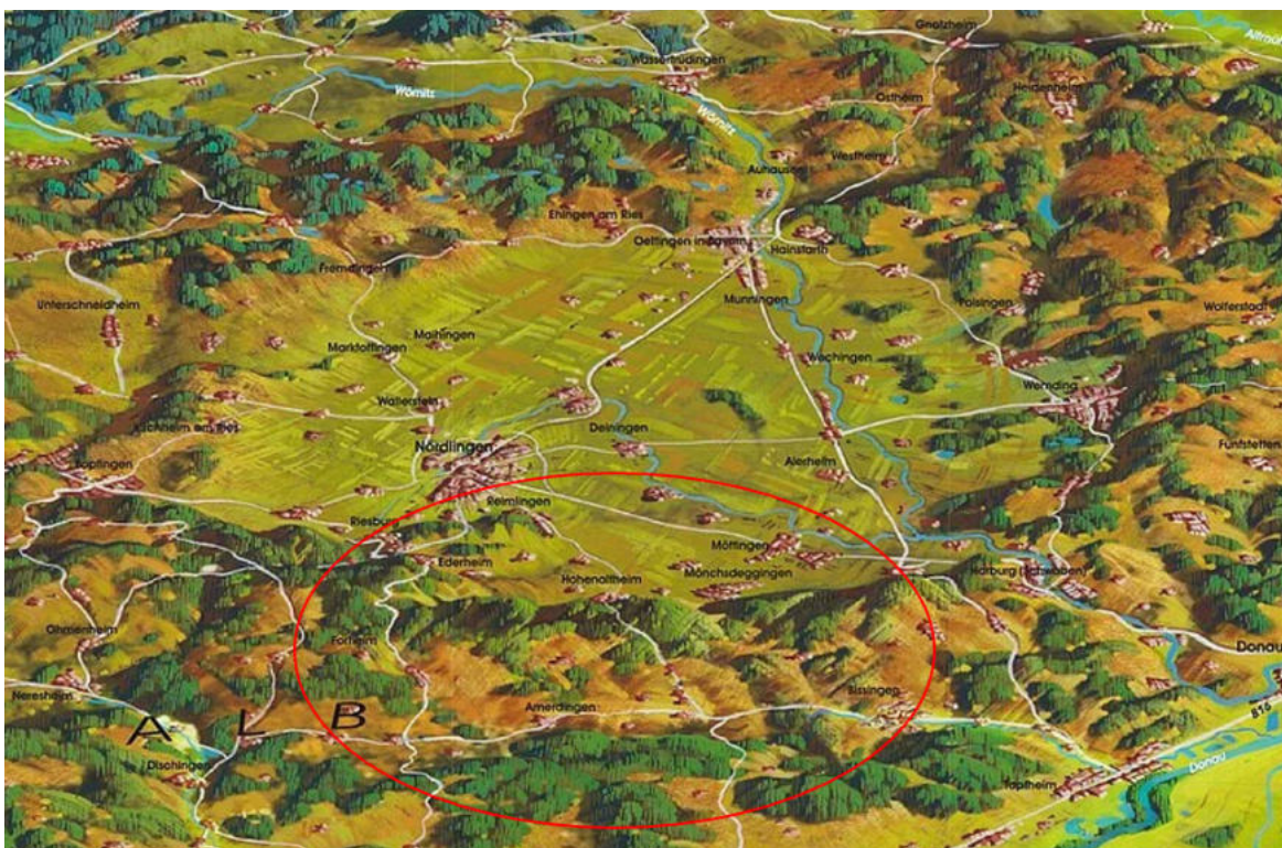
Abb. 32: Lage der ILE-Kommunen in und um den Rand des Rieskraters Quelle: Geopark Ries (bearbeitet)
